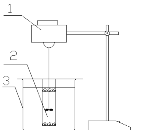
1—电动搅拌机; 2—有机玻璃筒; 3—实验缸
